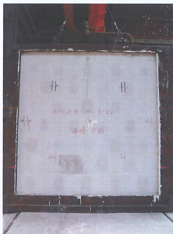
照片 6 加熱試驗後試體非曝火面
