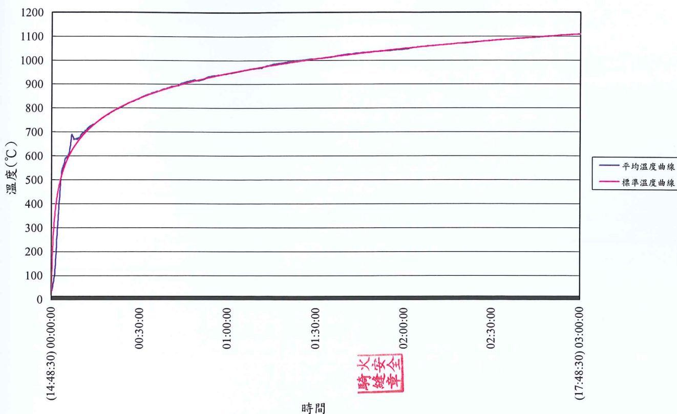
圖 4 爐內平均溫度曲線圖
